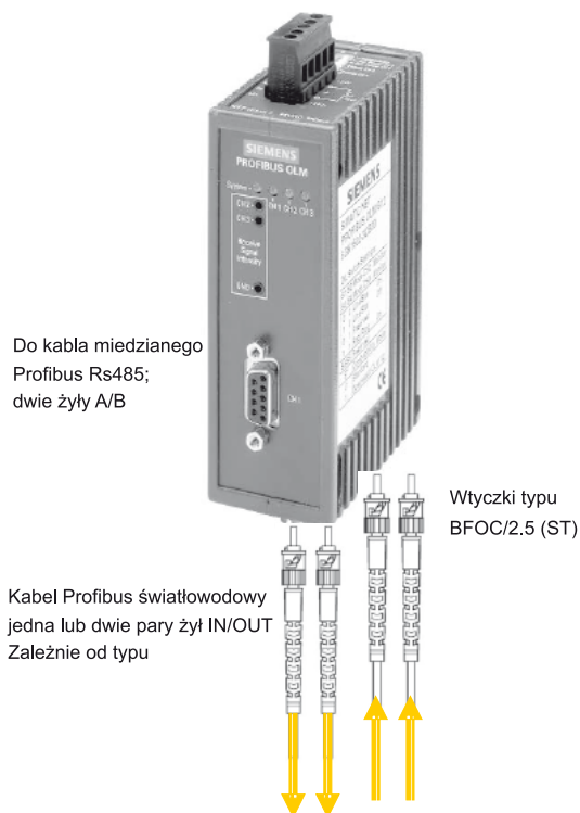
Fot. 4. Konwerter RS485/światłowod dla sieci Profibus
