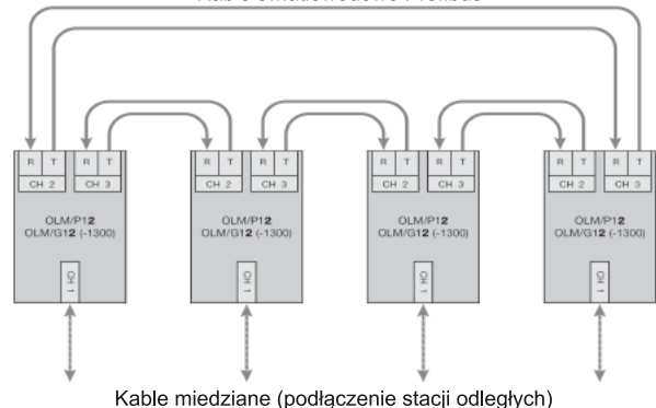
Rys. 3. Topologia pierścienia redundantnego w sieci Profibus
