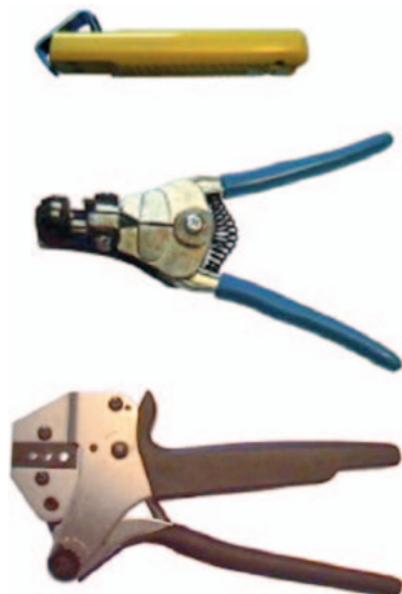
Fot. 7. Narzędzia do obróbki i zaciskania końcówek światłowodów BFOC oraz plastikowych
